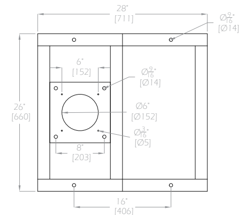
WSB-2400 Footprint
