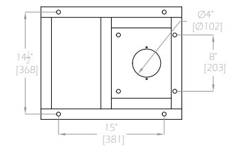
WSB-1860 Footprint
