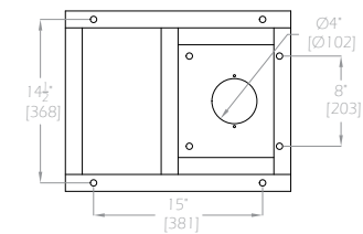
WSB-1840 Footprint
