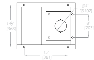
WSB-1820 Footprint
