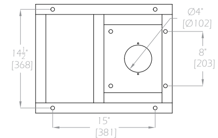
WSB-960 Footprint
