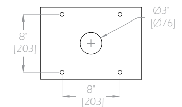
WSB-250 Footprint
