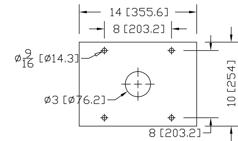
WSB 240 FOOTPRINT
