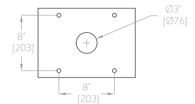
WSB-240 Footprint
