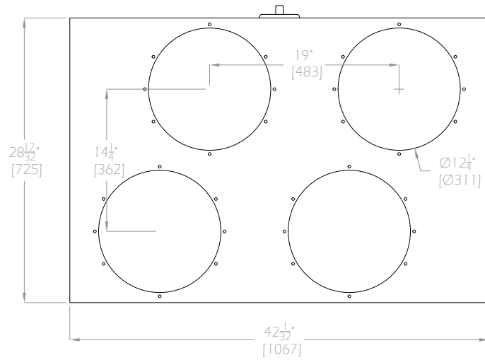
WSB-240 LID TOP VIEW
