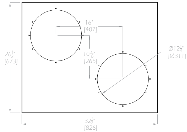
WSB-220 LID TOP VIEW
